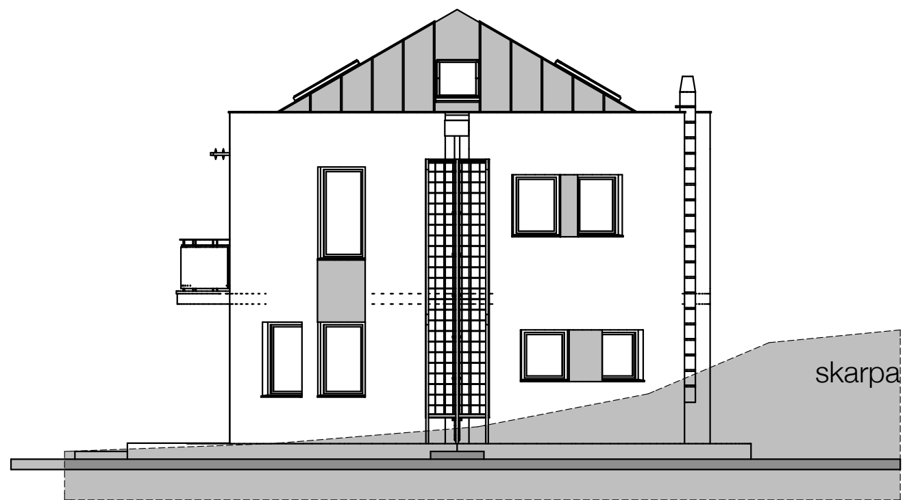
ELEWACJA BOCZNA
