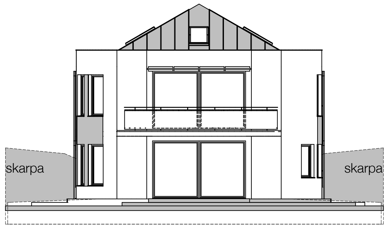
ELEWACJA FRONTOWA
