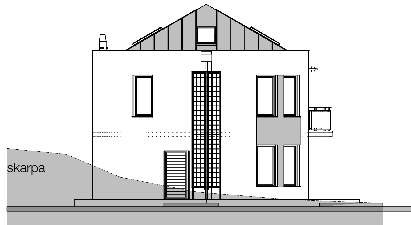
ELEWACJA BOCZNA
